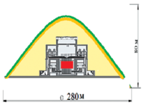
Рис. 1. Схема «зеленого кургану» над енергоблоком ЧАЕС
