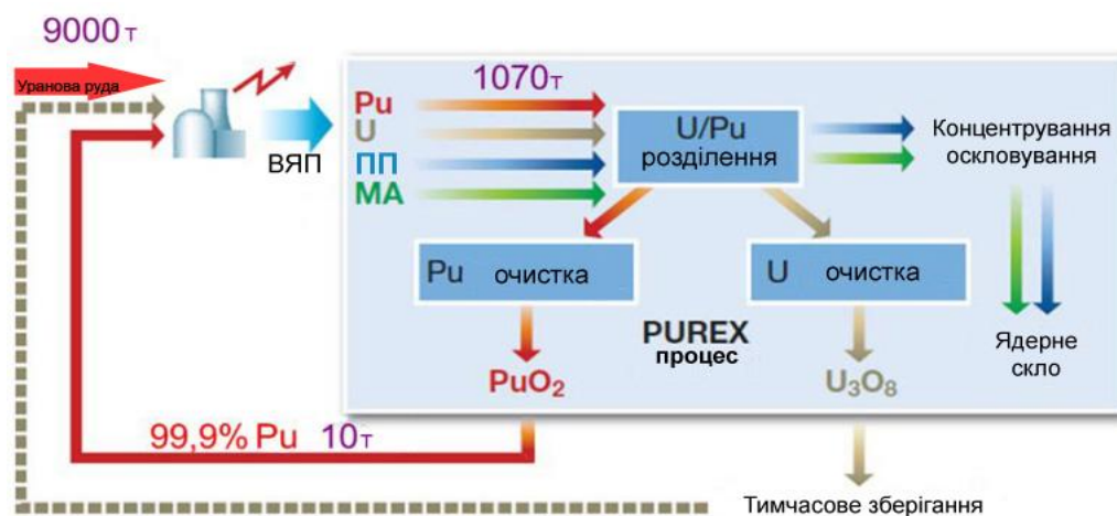
Рис. 2. Схема подвійного паливного циклу з використанням сепарації U, Pu, молодших актинідів і продуктів поділу (Франція) (адаптовано з [13]).
