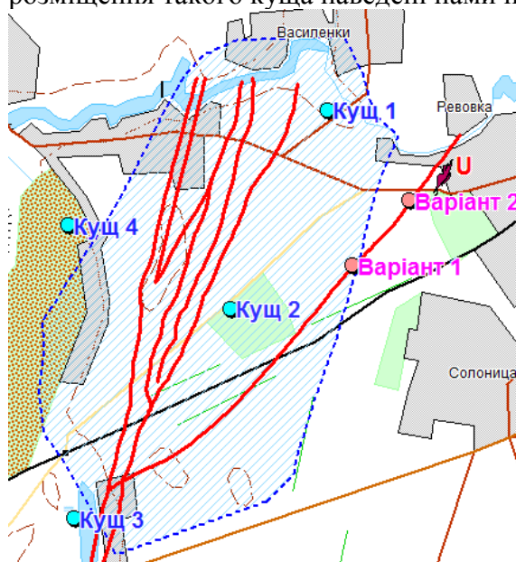
Рис. 2. Варіанти розміщення куща спостережних свердловин, який пропонується створити на Діагональному розломі в межах території Біланівського залізрудного та Кременчуцького уранового родовищ.
